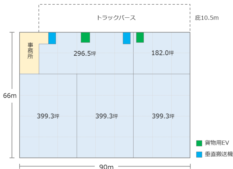
【配置図 (1階)】
