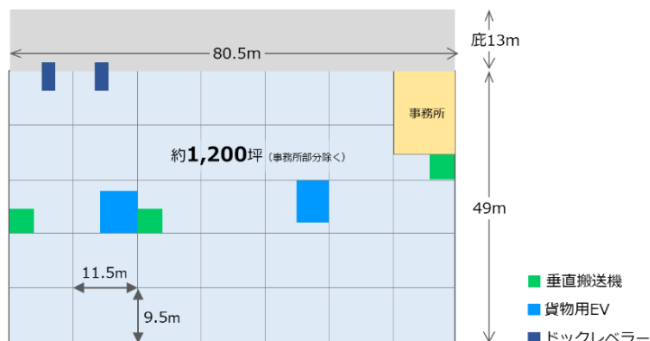
【配置図（1階）】
